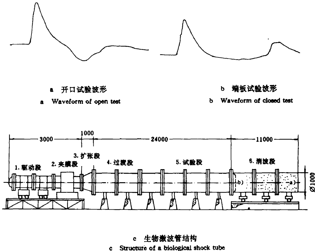
图1 生物激波管结构及波形因素
