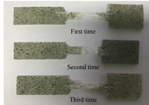
图 8 试件破坏图
