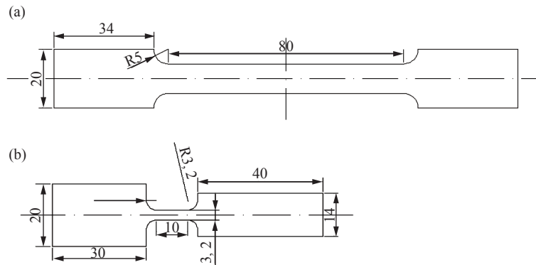
图 5 试件形状与尺寸 (单位: mm)
